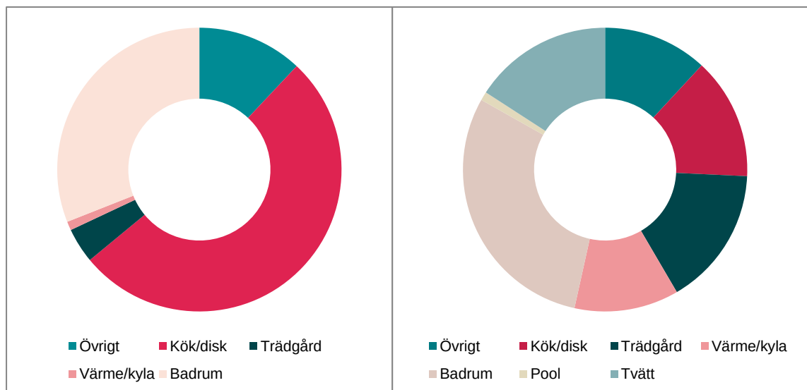
Figur 21. Vattenanvändning i amerikanska restauranger (vänster) och hotell (höger) (US EPA, 2012b).
