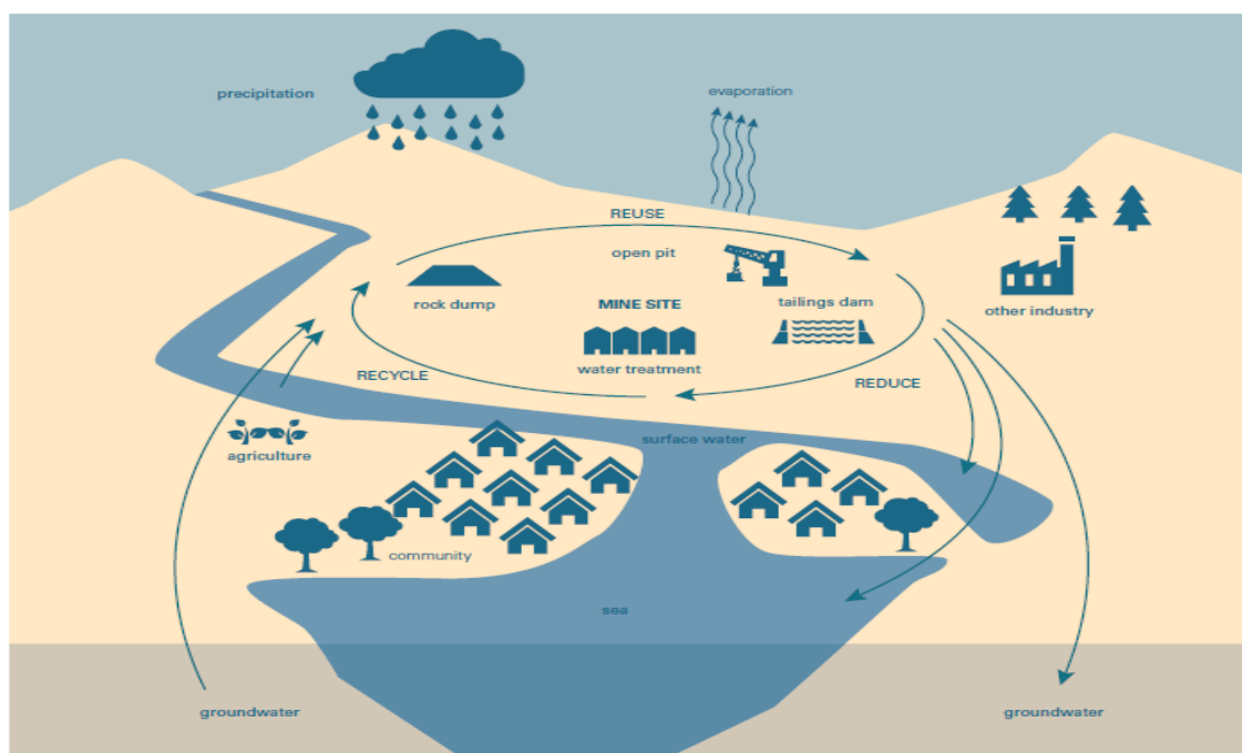
Figur 34. Typiska vattenflöden vid en gruva (Austrade, 2017; ICMM, 2012).
