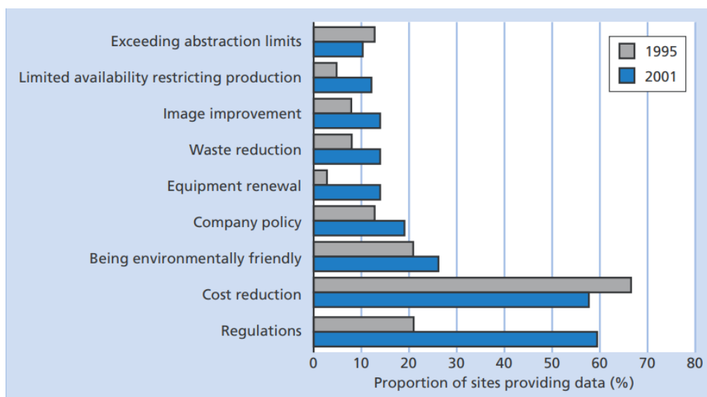
Figur 33. Drivkrafter för effektivare vattenanvändning i Storbritanniens pappers- och massaindustri (Envirowise, 2002).
